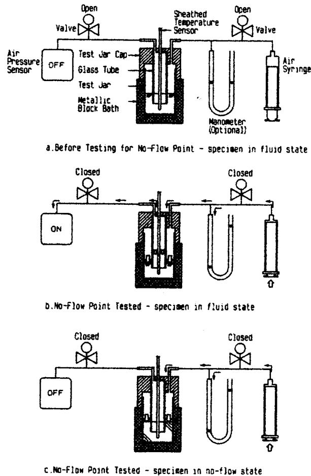
FIG. 1 Automatic Apparatus
