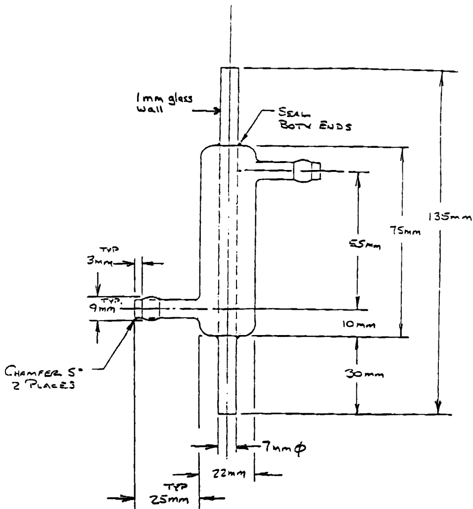
FIG. 2 Condenser
