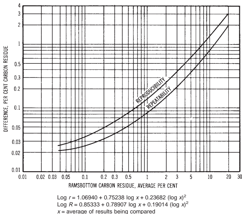
FIG. 4 Precision Data
