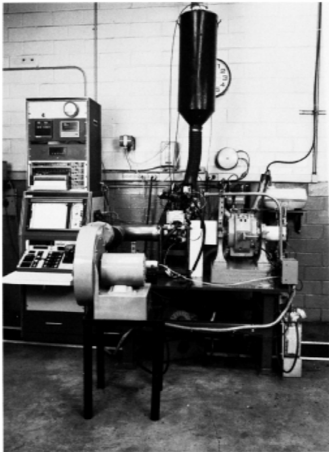
FIG. 1 Test Stand
