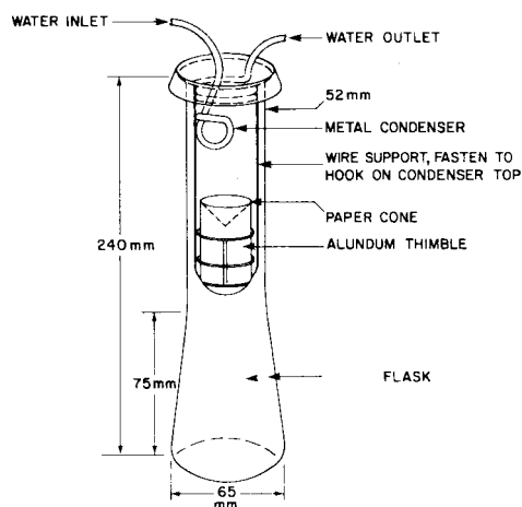
FIG. 1 Extraction Apparatus
